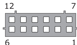
Рис. 3. Нумерация контактов в разьеме, вид со стороны проводов
