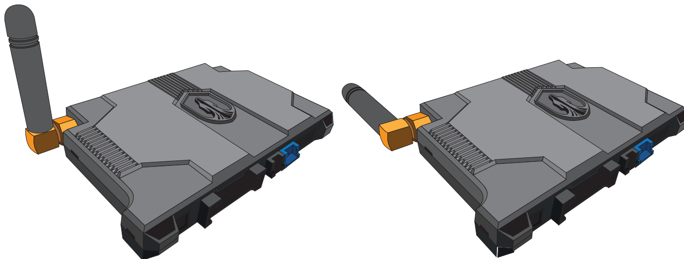
Рис. 1 Расположение GSM-антенны центрального блока сигнализации
