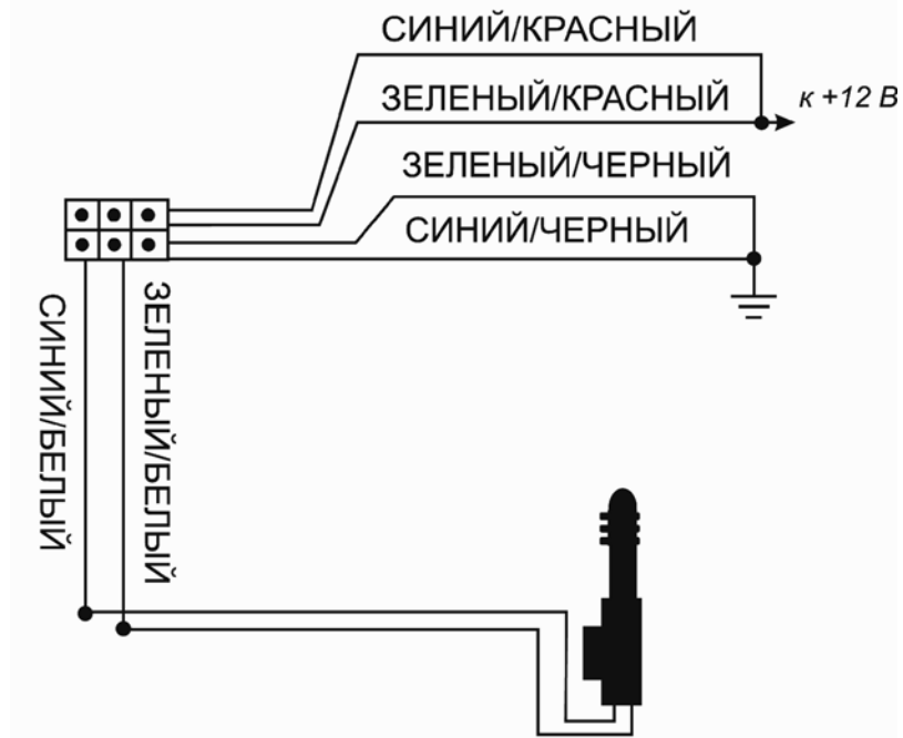
Схема 5 Установка дополнительных электроприводов
