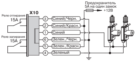
Схема подключения 2-проводных дверных замков с инверсией полярности
