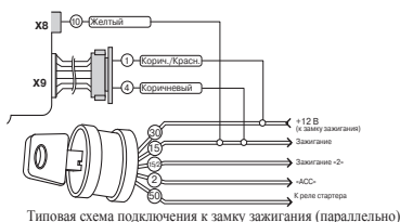
Типовая схема подключения к замку зажигания (параллельно)
