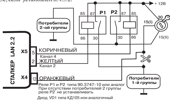
Рис. 14. Схема подачи зажигания при постановке на охрану с заведённым двигателем без ключа в замке зажигания
