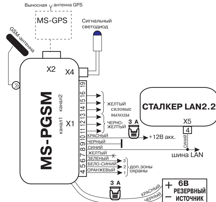
Рис. 21. Подключение MS-PGSM по шине LAN к охранному комплексу СТАЛКЕР LAN 2.2
