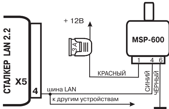
Рис. 19. Типовая схема подключения приемопередатчика MSP-600 к автомобильному охранному комплексу СТАЛКЕР LAN 2.2
