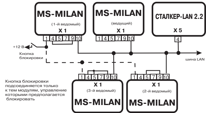
Рис. 17. Схема подключения модулей MS-MILAN
