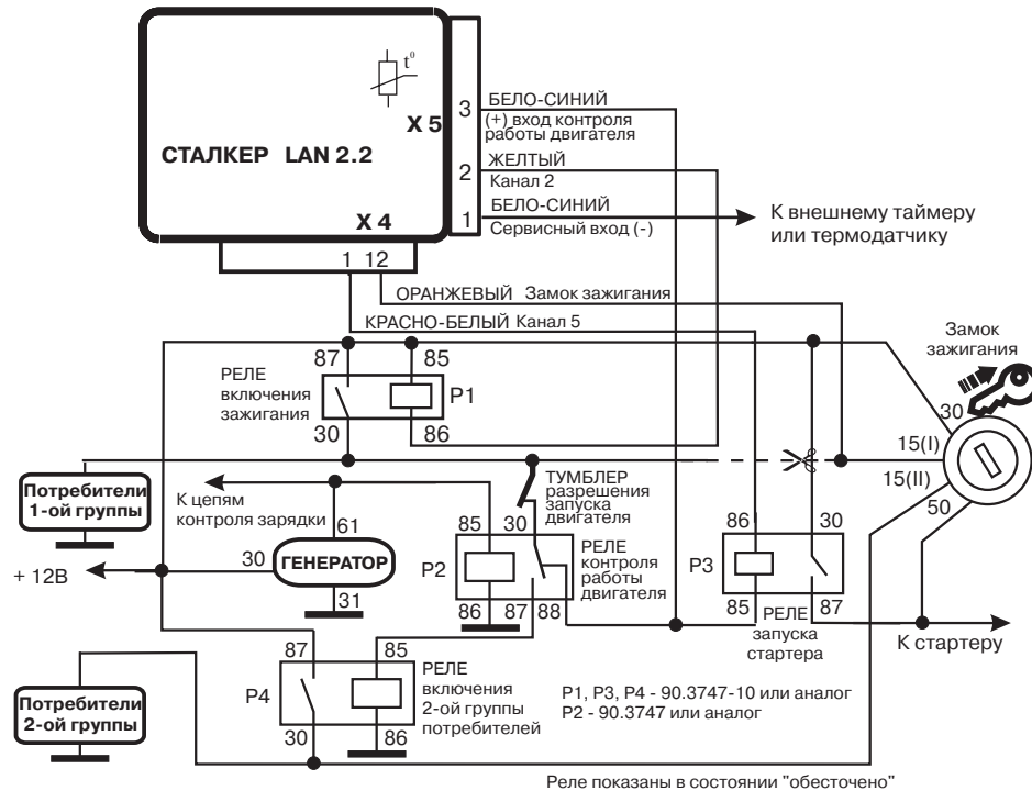
Рис. 10. Цепи дистанционного и автоматического запуска двигателя
