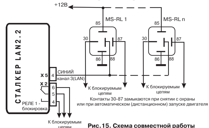
Рис. 15. Схема совместной работы комплекса СТАЛКЕР-LAN 2.2 и реле блокировки MS-RL
