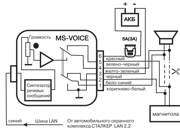
Рис. 18. Схема совместной работы комплекса СТАЛКЕР LAN 2.2 и синтезатора речевых сообщений MS-VOICE
