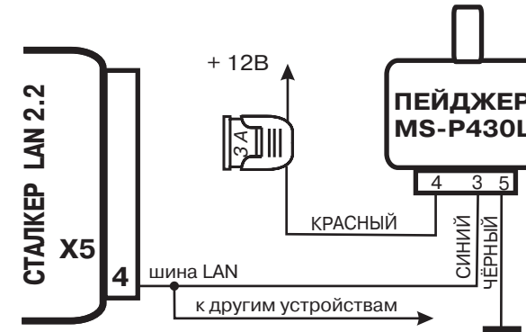
Рис. 20. Подключение пейджера MS-P430L, MS-P430L SUPER, MS-P430 SUPER N
