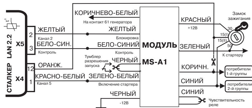
Рис. 11. Схема совместной работы охранного комплекса СТАЛКЕР LAN 2.2 и модуля дистанционного запуска MS-A1
