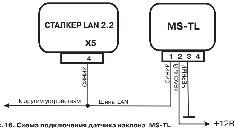
Рис. 16. Схема подключения датчика наклона MS-TL
