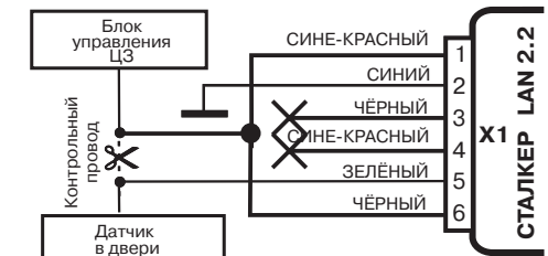
Рис. 8. Схема подключения к центральному замку, которому для отпирания требуется отрицательный импульс, а для запирания - разъединение проводов
