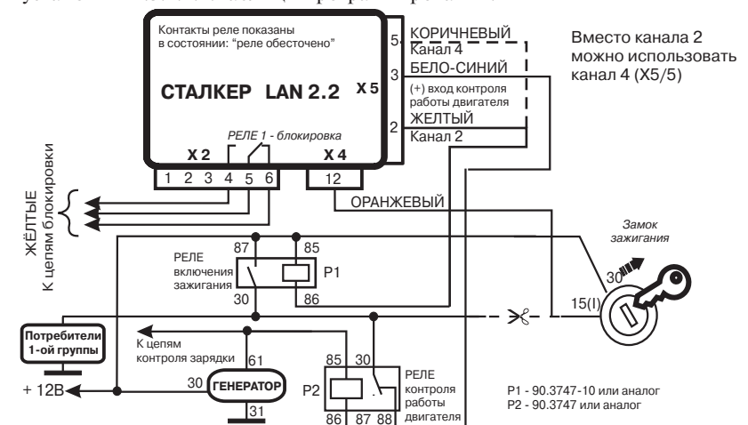
Рис. 13. Цепи для реализации режима "турбо"
