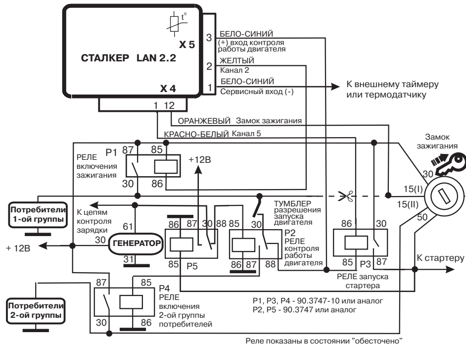
Рис. 12. Вариант схемы рис. 10 для случая отсутствия возбуждения генератора на холостых оборотах
