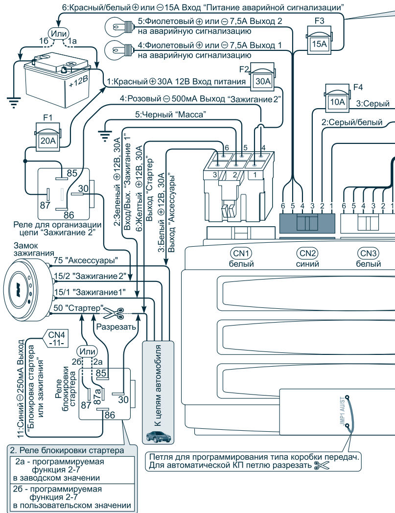
Схема 1
