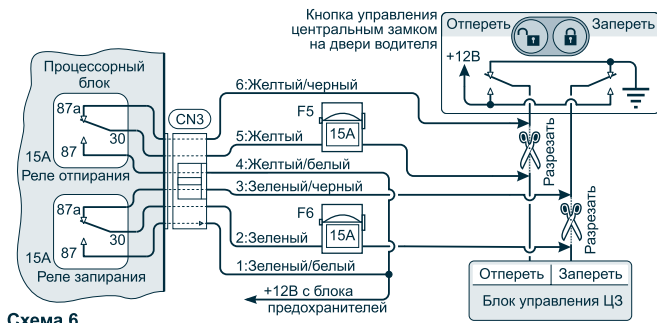
Схема 6
