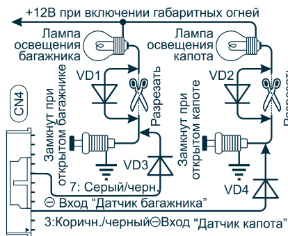
Схема 10
