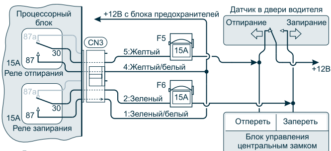
Схема 5
