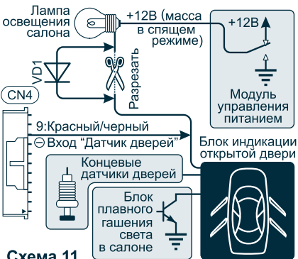
Схема 11
