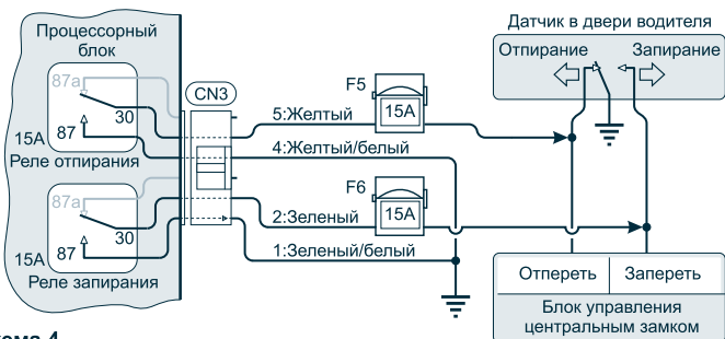
Схема 4
